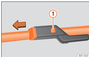
Sl. 158 Zamjena prednjih metlica brisača.
