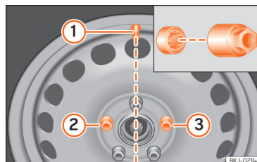
SL. 195 Zamjena kotača: ventil gume ① i mjesto ugradnje vijka kotača sa zaštitom od krađe ② ili ③.
