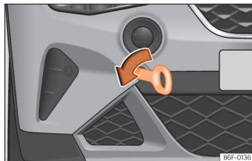
SL. 163 Prednji branik desno: zavrtnuta ušica za vuču
