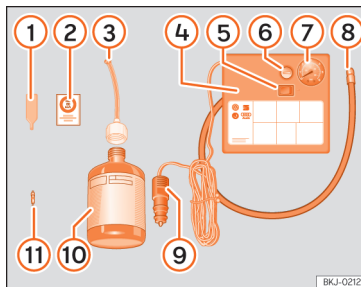
SL. 199 Prikaz principa: sastavni dijelovi kompleta za popravak guma
