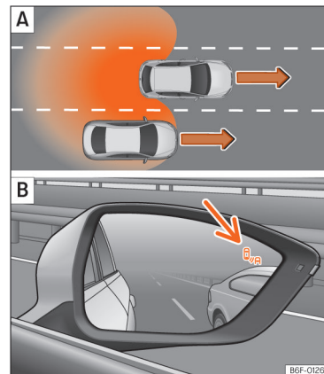
SL. 115 Shematski prikaz: A pretjecanje na srednjem voznom traku i povratak na desni kolnički trak. B Prikaz potpore pri promjeni voznog traka desno.
