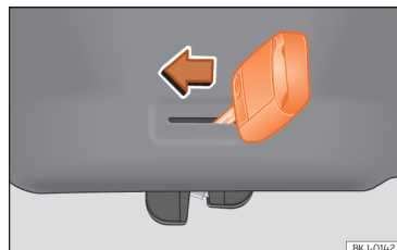
Sl. 58 Isječak iz prtljažnika: otključavanje u nuždi.
