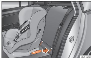
SL 38 Stražnja sjedala: ugradnja dječje sjedalice s ISOFIX sustavom.
