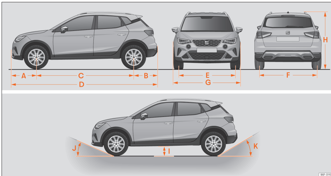
SL. 203 Dimenzije i kutevi.
