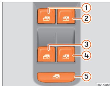
Sl. 59 Isječak iz vozačevih vrata: tipke za rukovanje električnim podizačima prozora
