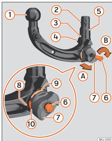
Sl. 152 Pregled: mehanizam za vuču s mogućnošću skidanja
