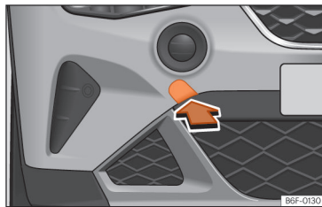
SL. 162 Na desnoj strani prednjeg branika: skidanje poklopca.
