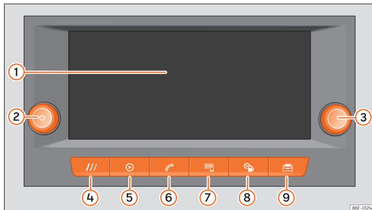
Sl. 136 Općeniti pregled: Jedinice za rukovanje i prikaz u izvedbi 8,25 inča.
