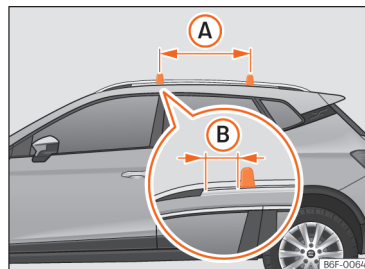
Sl. 147 Pričvrstne točke uzdužnih nosača za krovni nosač prtljage
