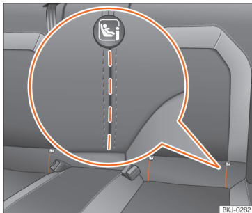
SL 37 Stražnje sjedalo: urezani prorezi za pristup ISOFIX/i-Size pričvršnim ušicama.
