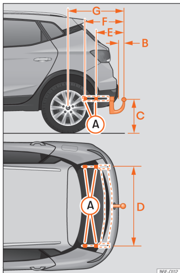
Sl. 151 Dimenzije i pričvrstna mjesta za naknadnu ugradnju mehanizma za vuču
