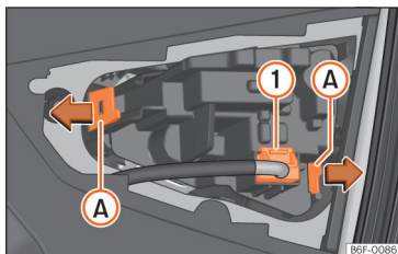
SL. 172 Demontaža držača žaruljice.
