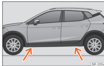
SL. 196 Mjesta za postavljanje dizalice vozila.
